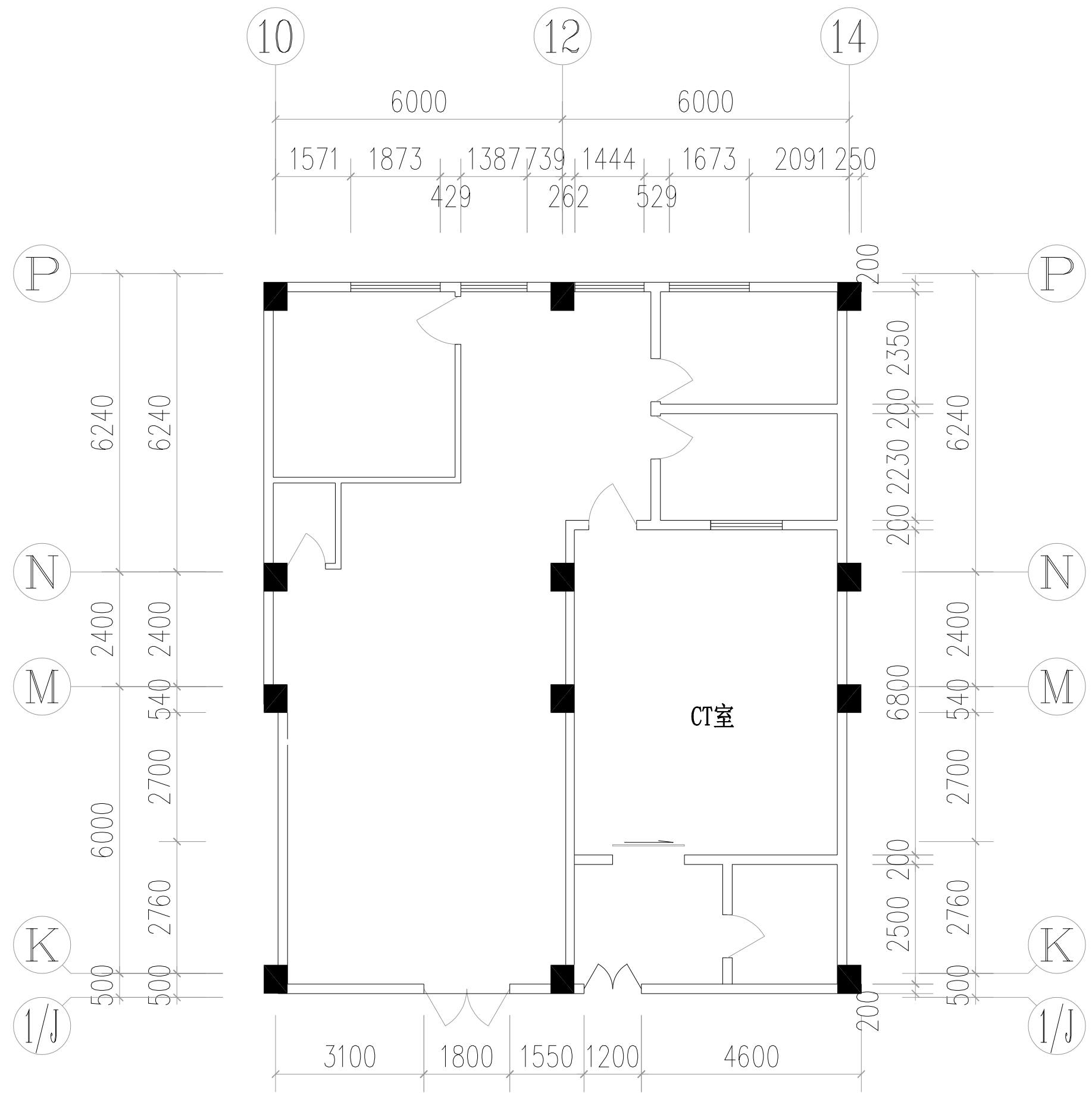
改造后图纸
